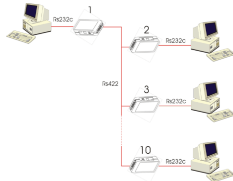
Schema di collegamento converter Rs232c/Rs422
