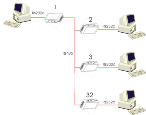
Schema di collegamento converter Rs232c/Rs485
