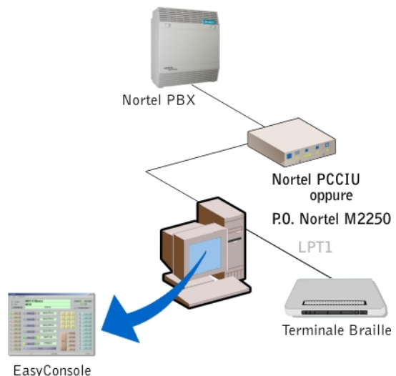
Schema di collegamento con sistema Nortel PCCIU o P.O. Nortel M2250
