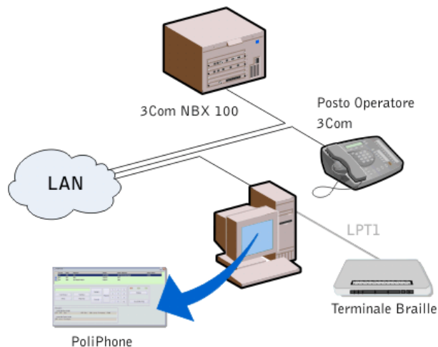
Schema di collegamento TAPI con sistema 3Com® NBX 100
