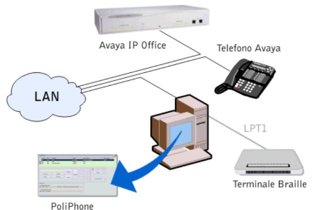
Schema di collegamento TAPI con sistema Avaya® IP Office
